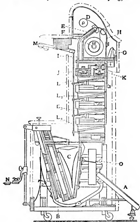
FIG. 36.—Modern Pianola.
