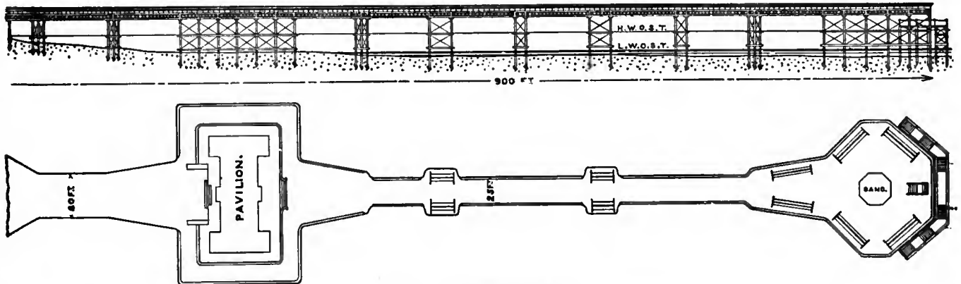
FIG. 3.—Promenade Pier.
