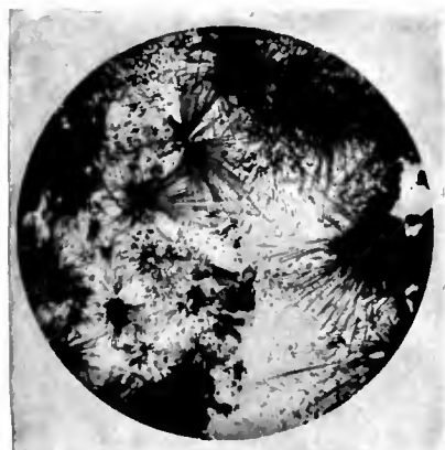
FIG. 7.—LUXULLIANITE, LUXULYAN, CORNWALL ( \times 15 ).
