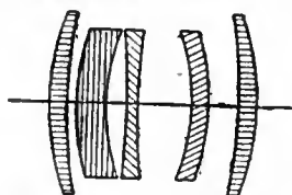
FIG. 55.—Beck's "Isostigmat."
