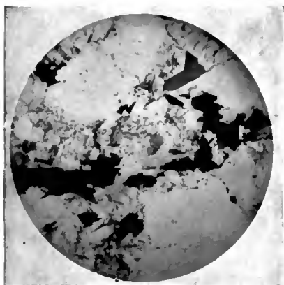
FIG. 4.—GRANITE RUBISLAW, ABERDEEN ( \times 10 ).
