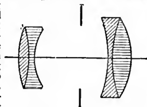
FIG. 58.—"Bis-Telar."
