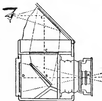
FIG. 10.—Reflex Camera.
