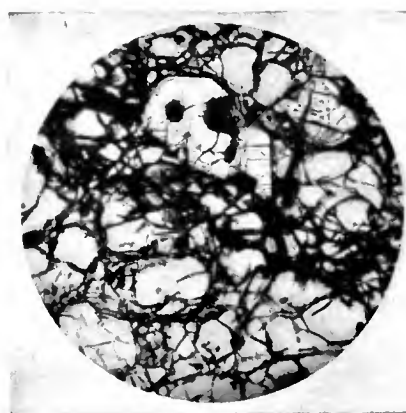
FIG. 5.—PERLITIC PITCHSTONE, MEISSEN, GERMANY ( \times 15 ).
