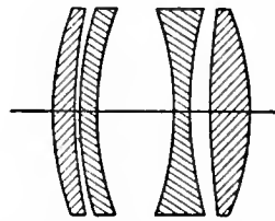
FIG. 43.—Planar. Series Ia. f/4 . FIG. 44.—Zeiss's "Unar."
